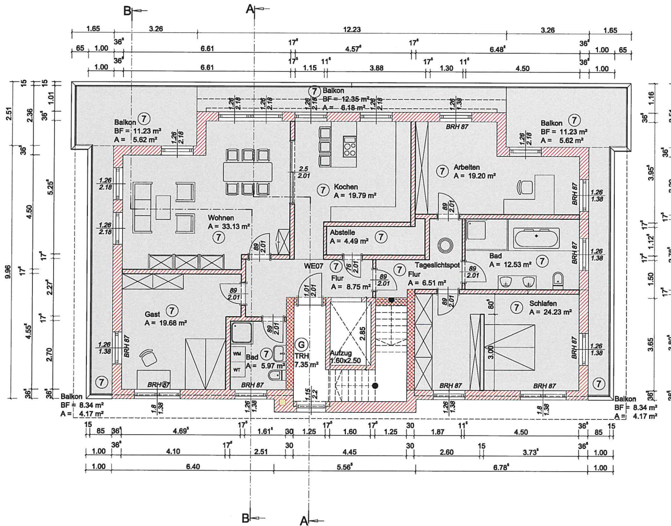
Grundriss - 3.OG
