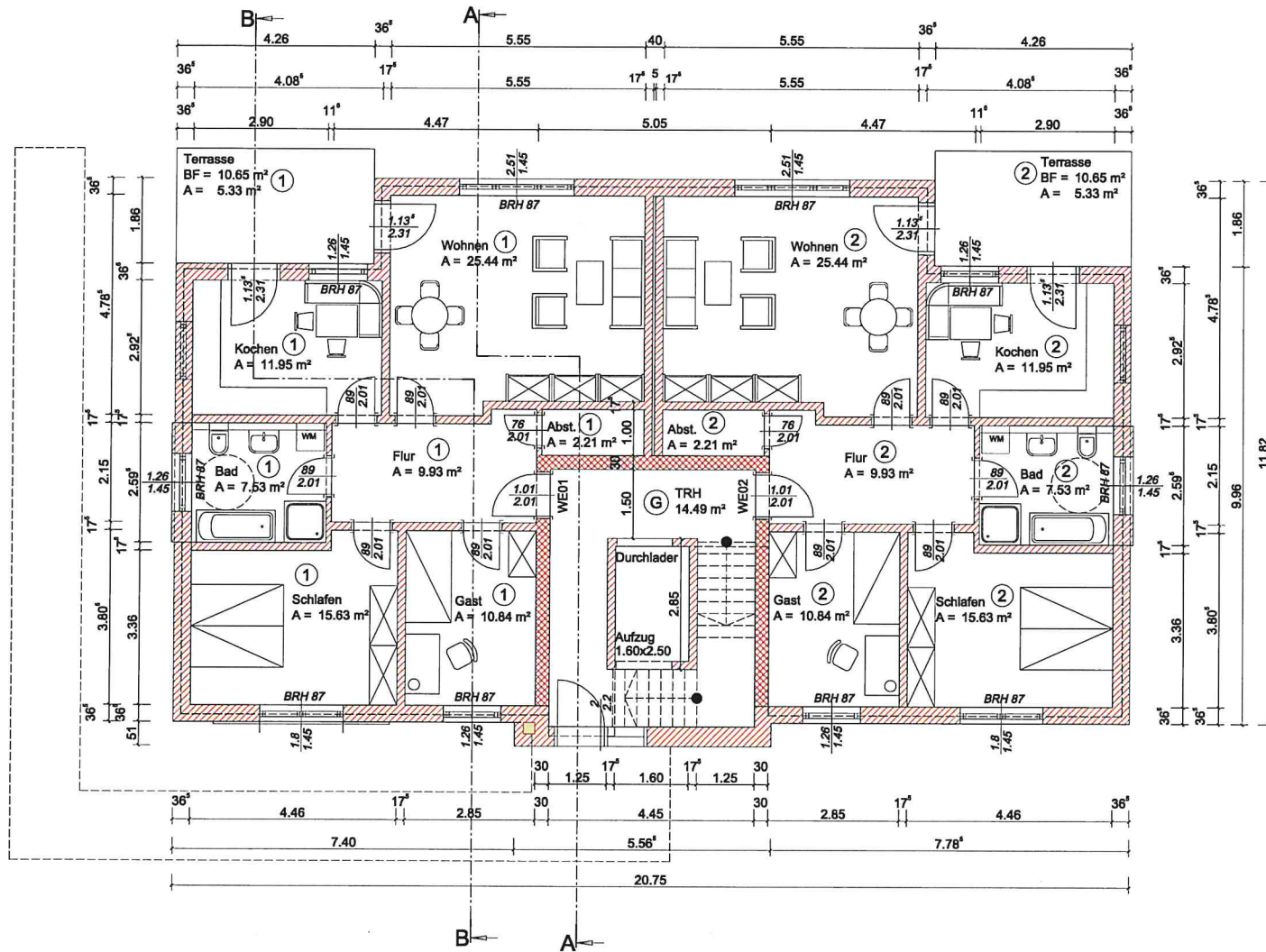
Grundriss - EG
